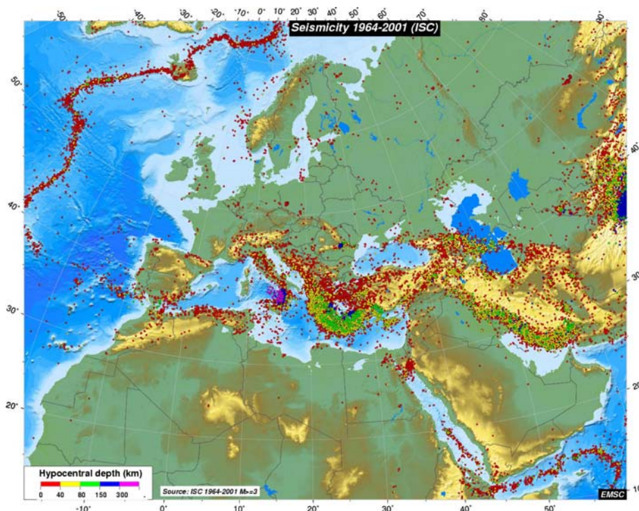
Mapa 2.34. Sismicitat 1964-2001 (Font: EMSC)
