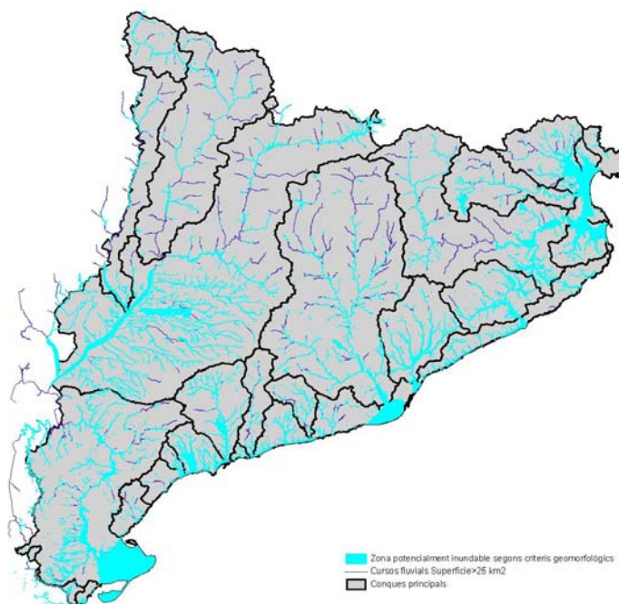
Mapa 2.9. Representació per conques hidrogràfiques principals de la informació existent de les zones potencialment inundables segons criteris geomorfològics.
